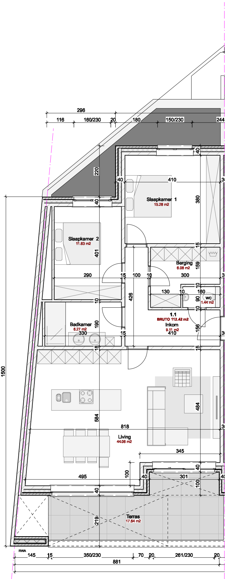
niv 01 - appartement 1.1 schaal 1/100
