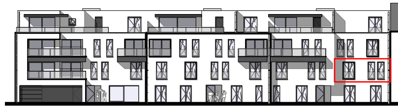
voorgevel
